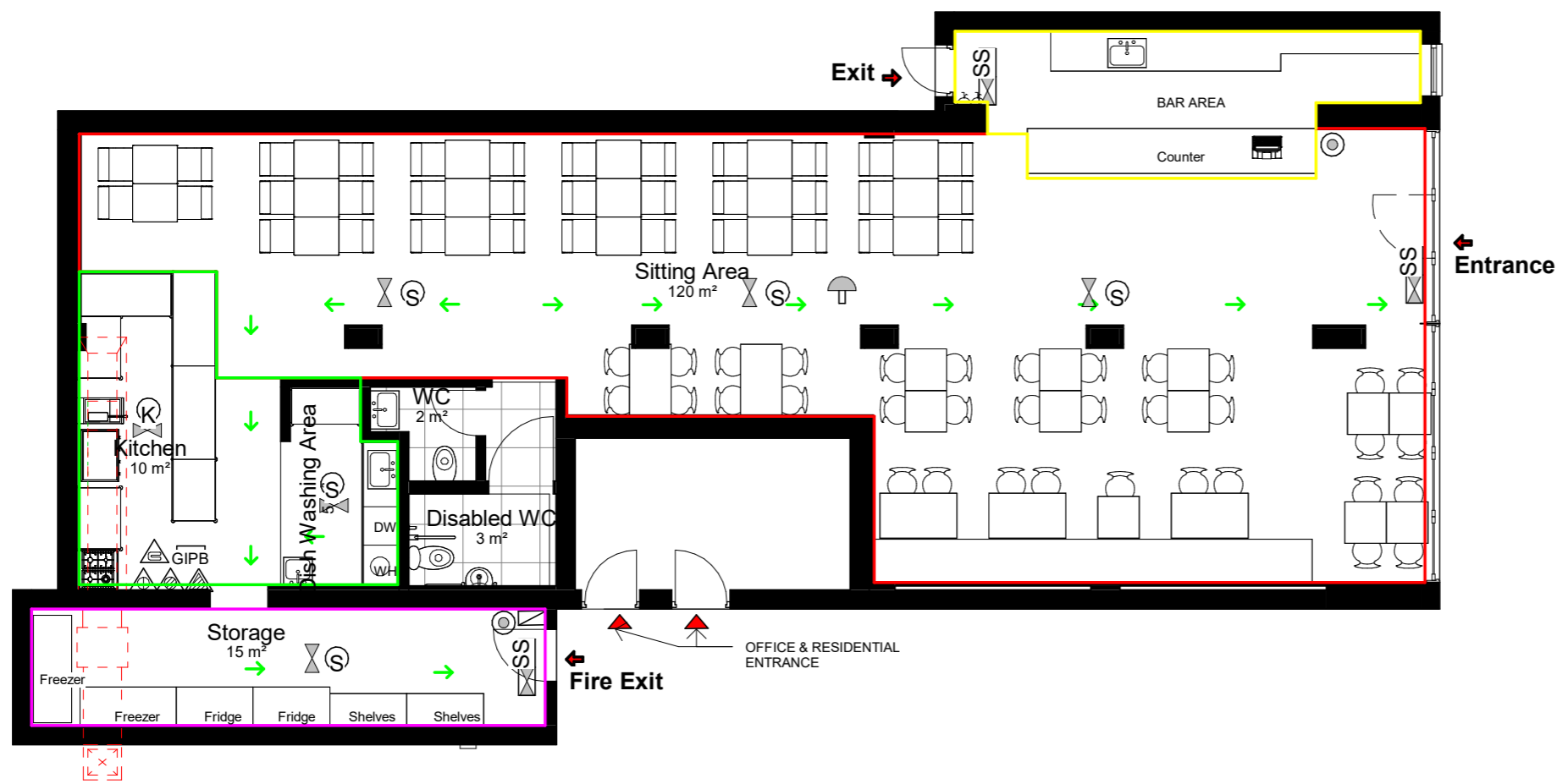
1 Floor Plan 1 : 100
